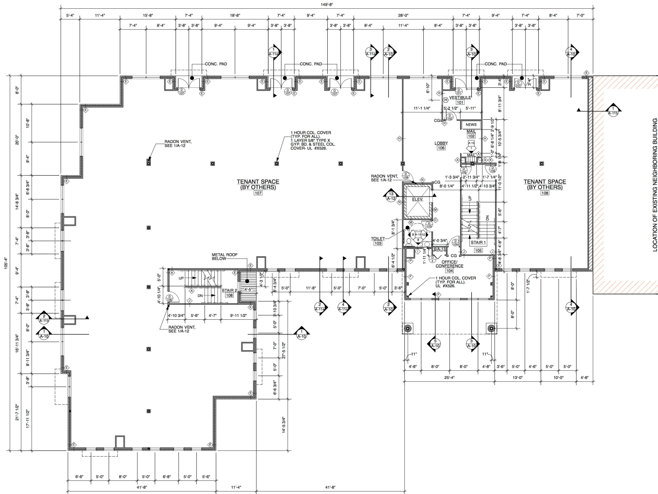
1 FIRST FLOOR PLAN A-3 SCALE: 1/8" = 1'-0"
