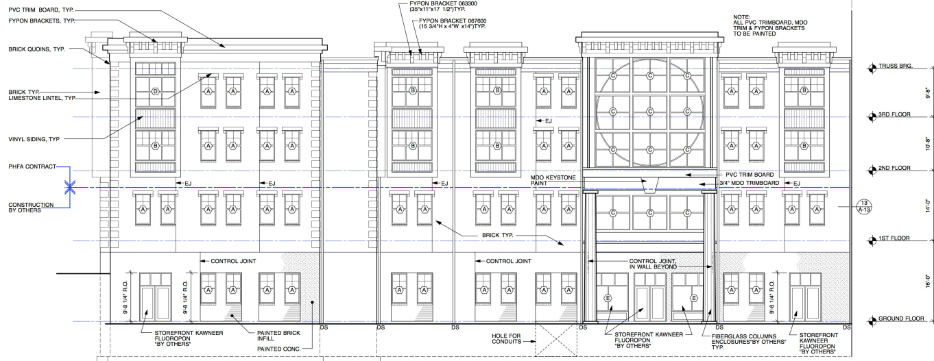
1 SOUTH ELEVATION SCALE: 1/8" = 1'-0"
