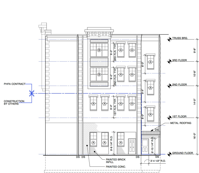
3 EAST ELEVATION SCALE: 1/8" = 1'-0"
