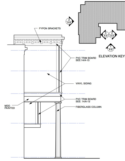
2 WEST ELEVATION SCALE: 1/8" = 1'-0"
